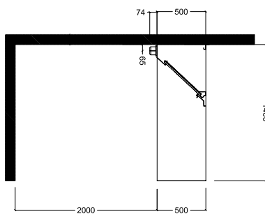
Zij aanzicht
